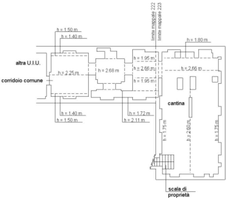
PIANO PRIMO SOTTOSTRADA (PS1)
